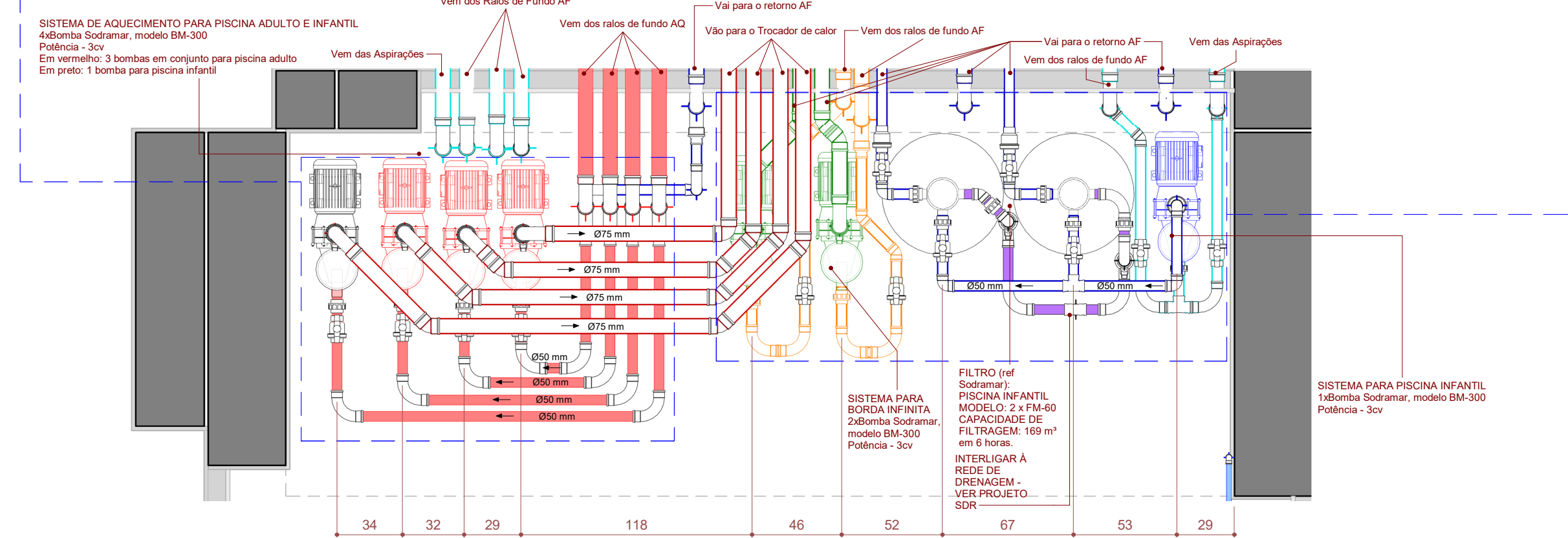
PLANTA BAIXA - CASA DE MÁQUINAS SUPERIOR ESCALA 1:25
