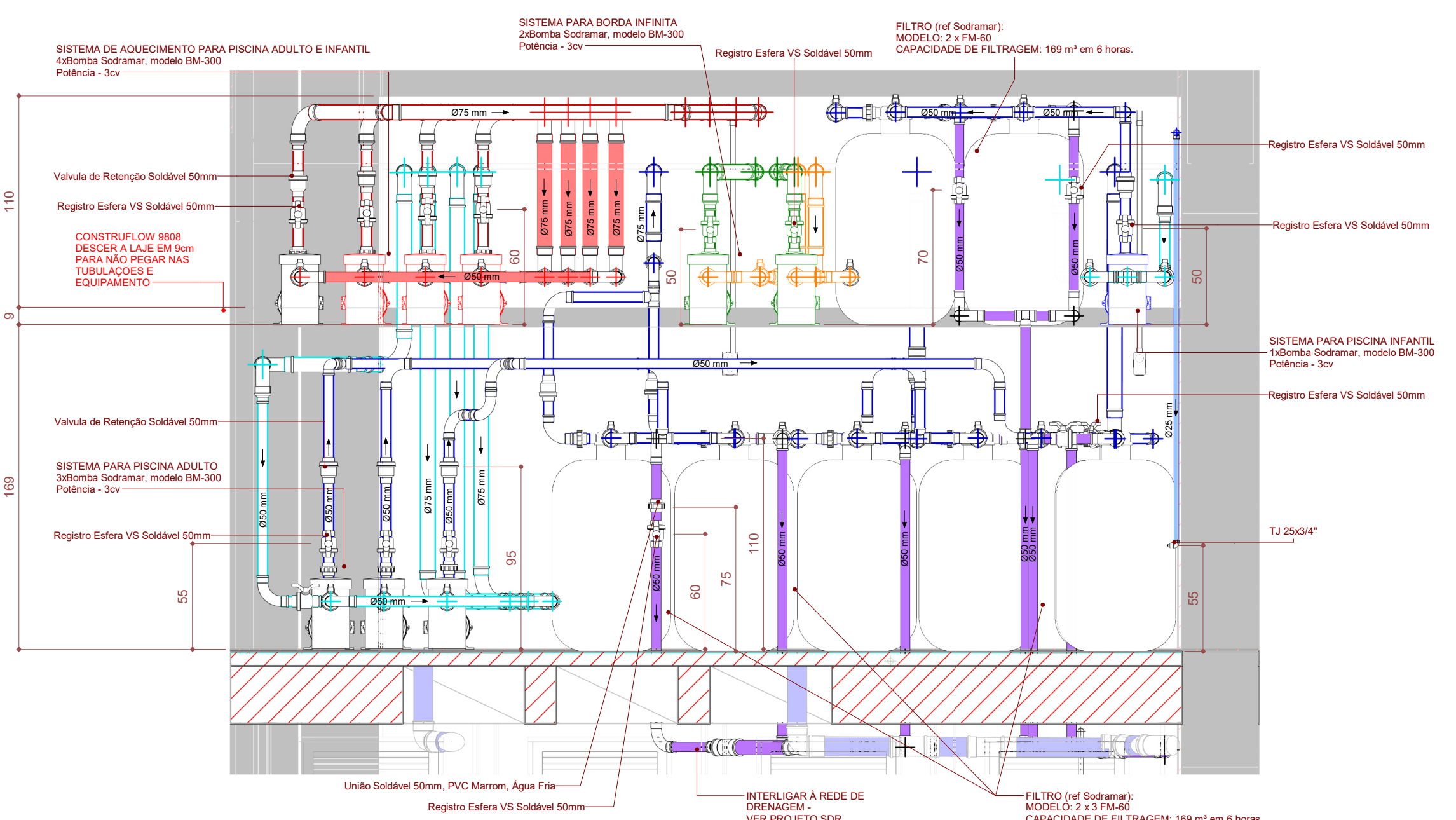
CORTE - CASA DE MÁQUINAS ESCALA 1:25
